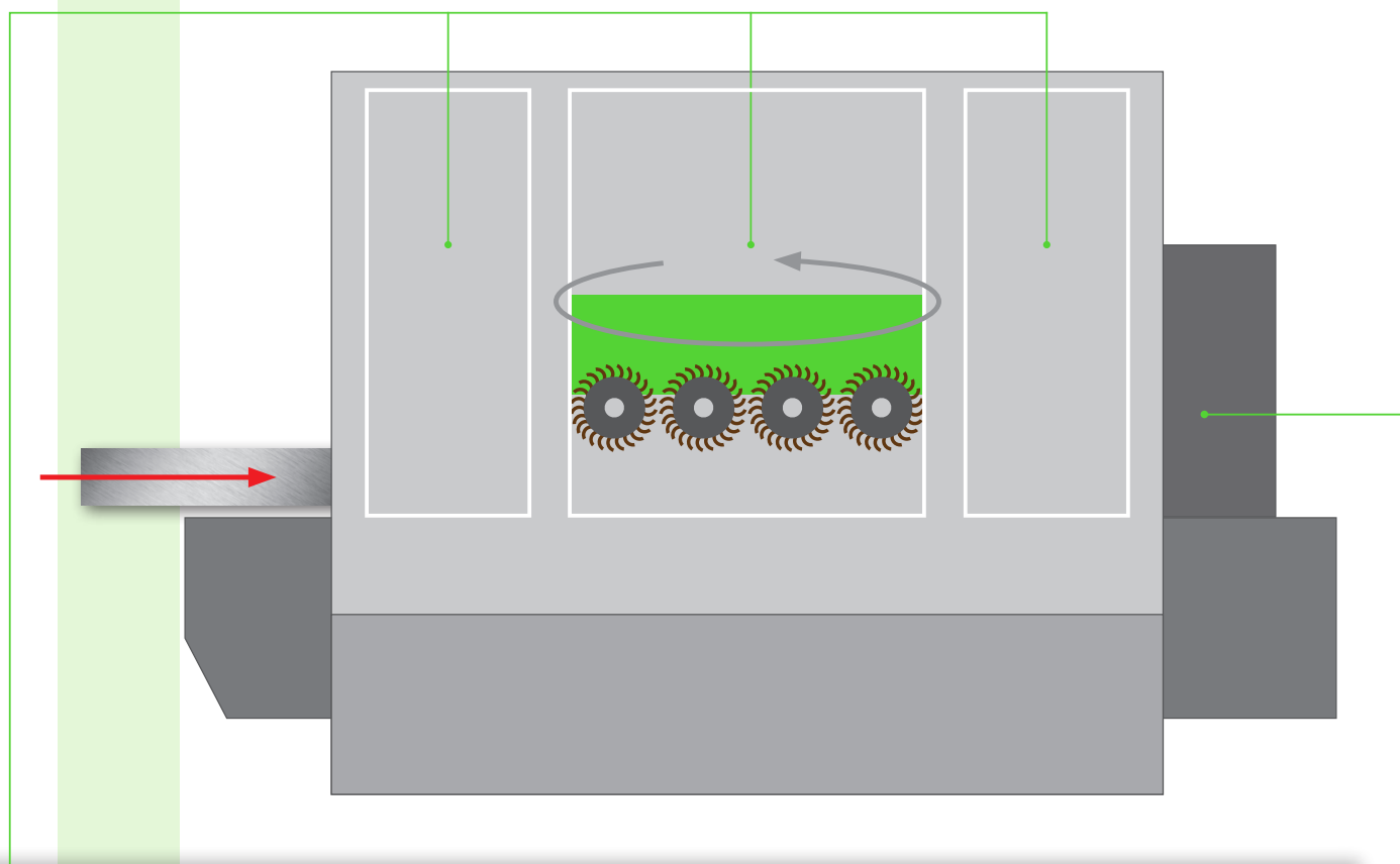
12B Sistema di lavoro planetario con 12 spazzole rotanti Planetary working system by 12 brushes Sistema de trabajo planetario por 12 cepillos
